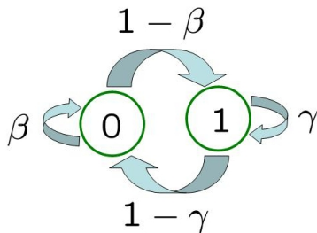
Fig. 5. Gilbert-Elliott Model
